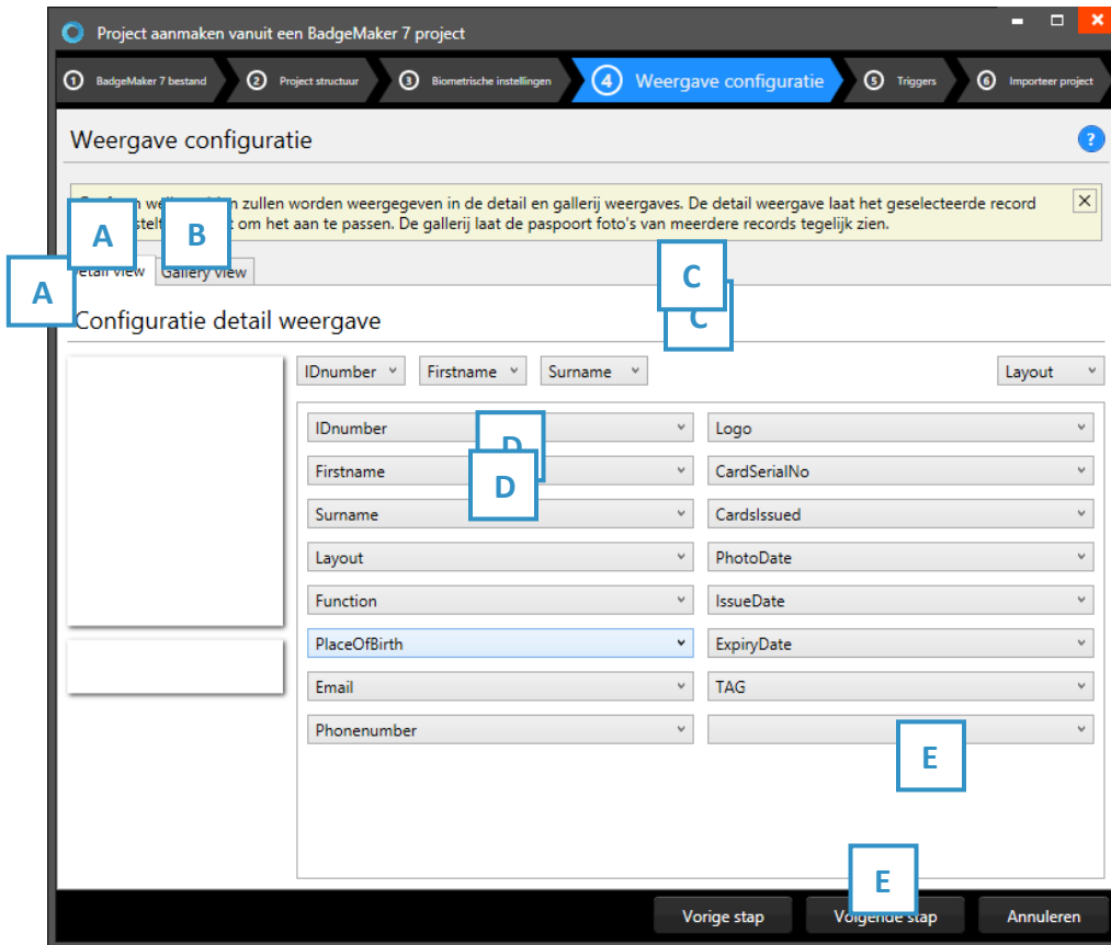
Fig. Voorbeeld van stap 4. Nieuw project: Weergave configuratie
