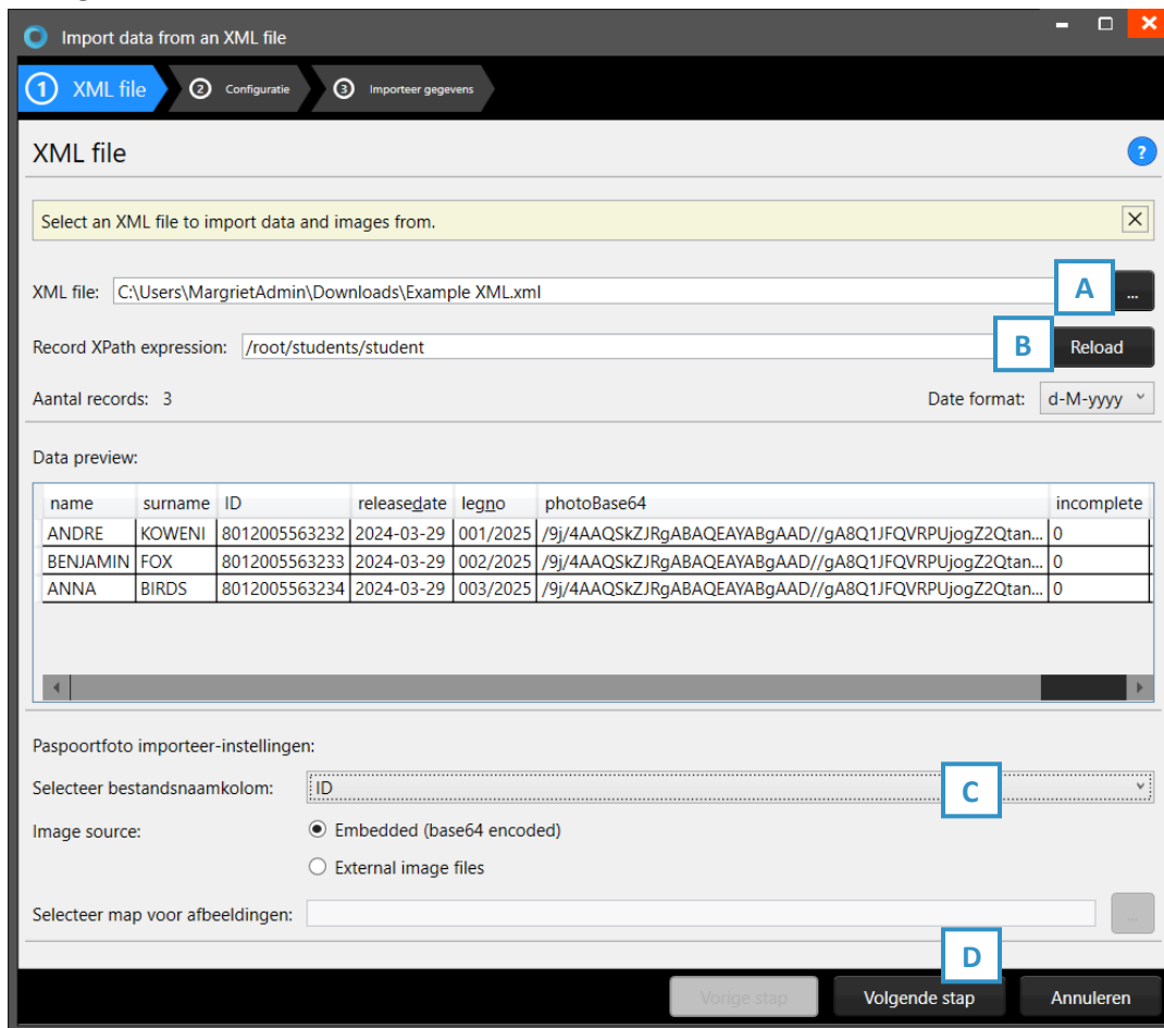
Fig. Voorbeeld van het pop-upvenster voor het importeren van gegevens Stap 1. Selecteer het XML-bestand.
