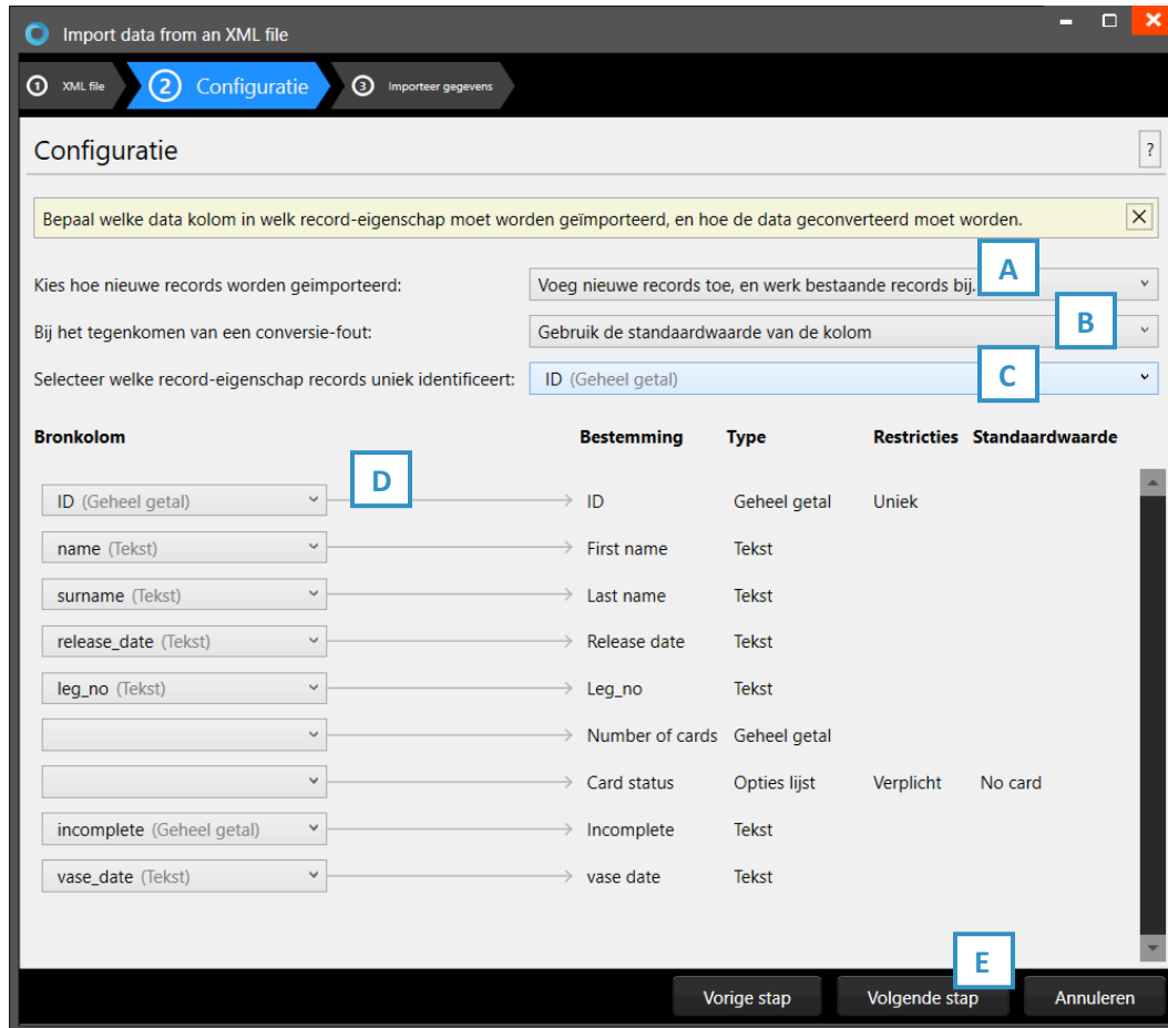
Fig. Voorbeeld van het pop-upvenster voor het importeren van XML-gegevens: Stap 2. Configuratie.
